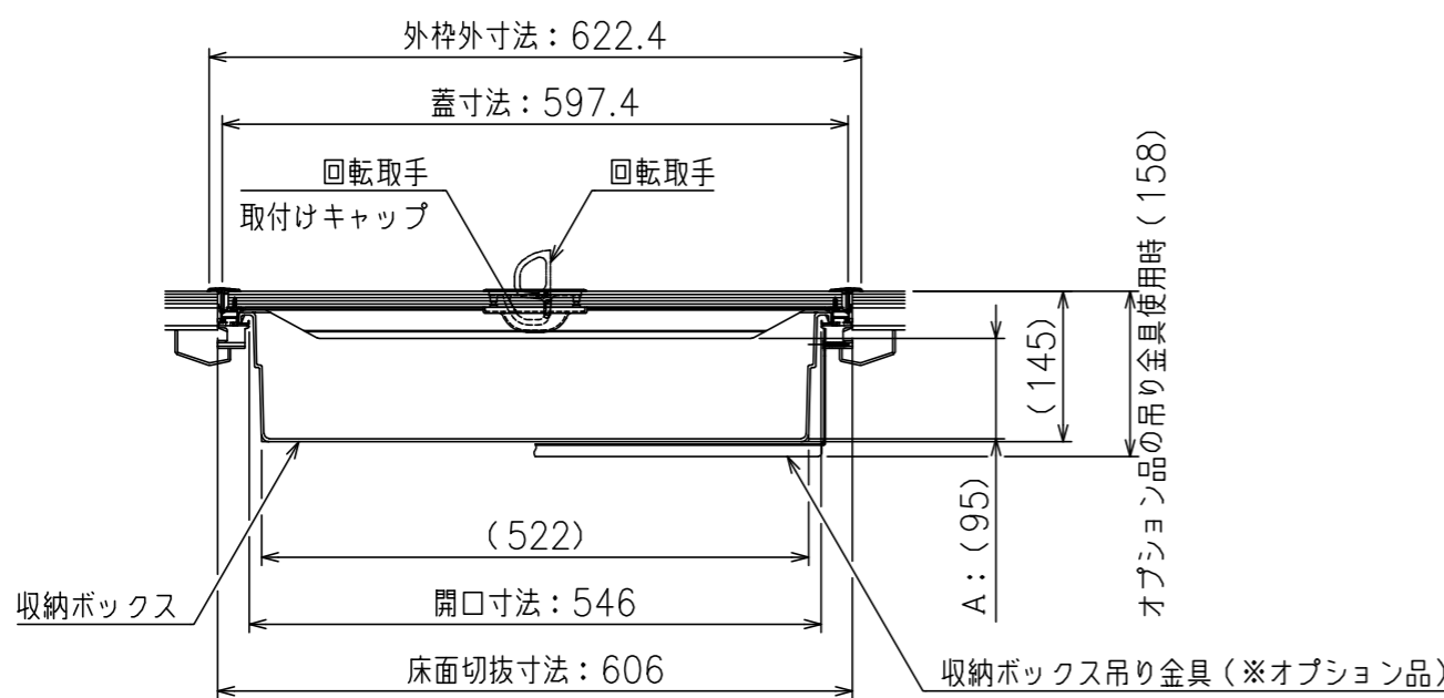
AA断面 1:8
